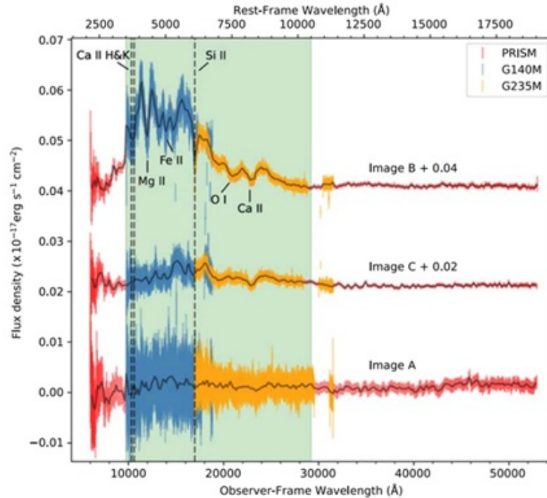
Gambar 6: Spektrum SN H0pe yang diamati dengan instrumen NIRSspec G140M, G235M, dan PRISM (Chen et al. [2024]).
