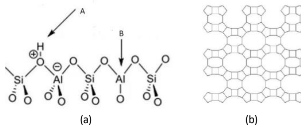
Gambar 1. Ion silikat dan aluminat (a) pada kerangka zeolit mordenite (b)
